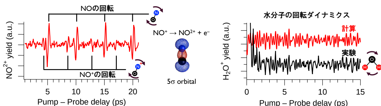
(左) 高強度光によって誘起された NO, NO + の回転運動の実時間計測結果 高強度光による NO + から NO 2+ の生成は 5σ軌道からのイオン化であることを明らかにした (右) 高強度光によって誘起された H 2 O 分子の複雑な回転運動
