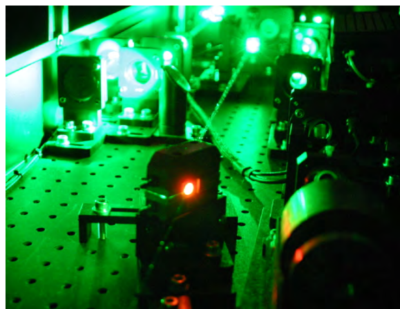
チタンサファイア再生増幅器
